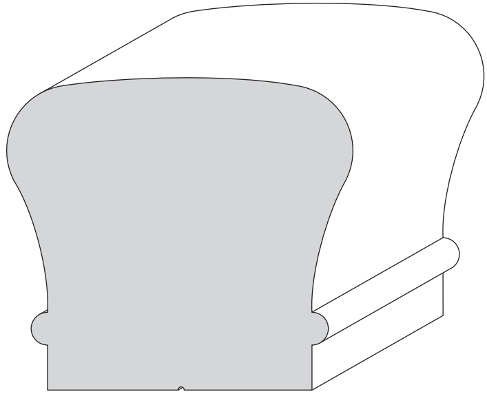
6210 2 3/8 x 2 5/8
